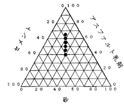
図-1 三角座標による配合分布図
