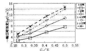
図-2 一軸圧縮強度とC/Eの関係(砕石1)
