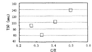
図-7 T50における緩和時間(砕石1)
