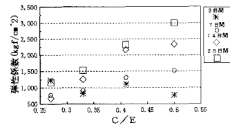
図-5 弾性係数とC/Eの関係(砕石1)
