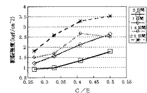
図-3 割裂強度とC/Eの関係(砕石1)
