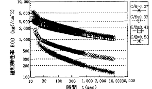
図-6 緩和弾性率と時間の関係(砕石1)
