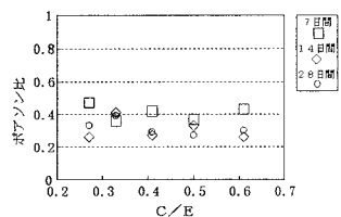
図-4 ポアソン比とC/Eの関係(砕石2)
