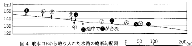
図4 取水口Bから取り入れた水路の縦断勾配図
