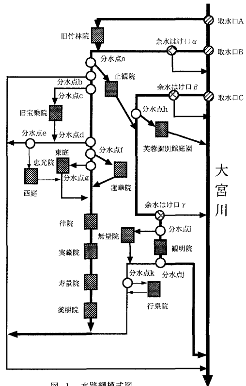
図1 水路網模式図
