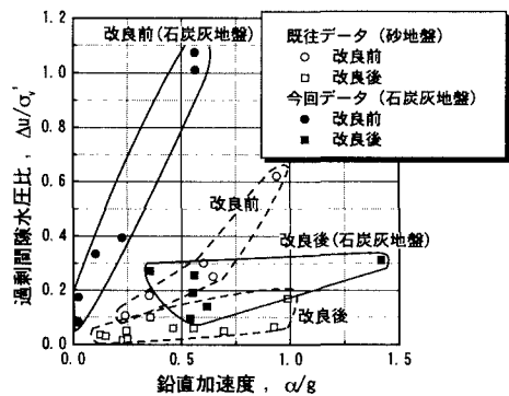
図-5 現位置液状化試験結果
