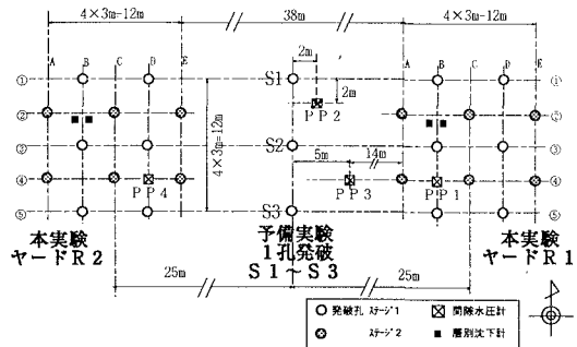
図一1 発破孔および計測位置平面図
