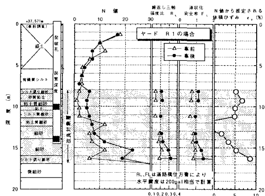
図一2 地盤条件および改良効果の確認
