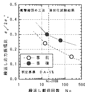
図-3 液状化強度試験結果
