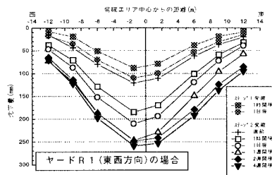
図-5 地表面沈下量分布図
