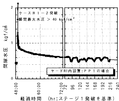
図-5 間隙水圧の経時変化
