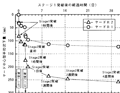
図-4 地表面沈下の経時変化
