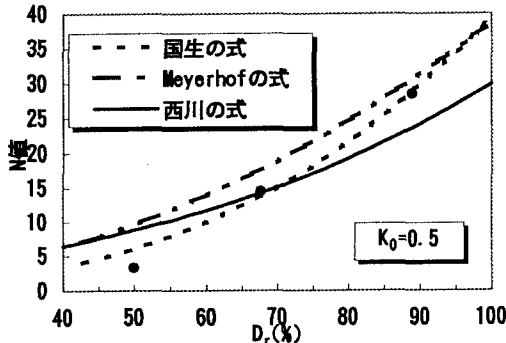
図2 K_0=0.5 におけるN値- D_r 関係
