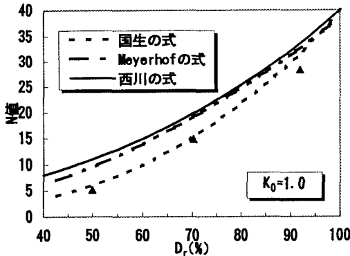
図4 K_0=1.0 におけるN値- D_r 関係
