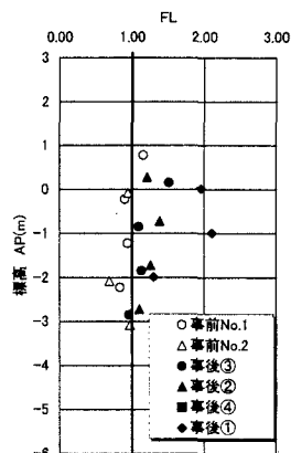
図-5 改良前後のFL値の比較
