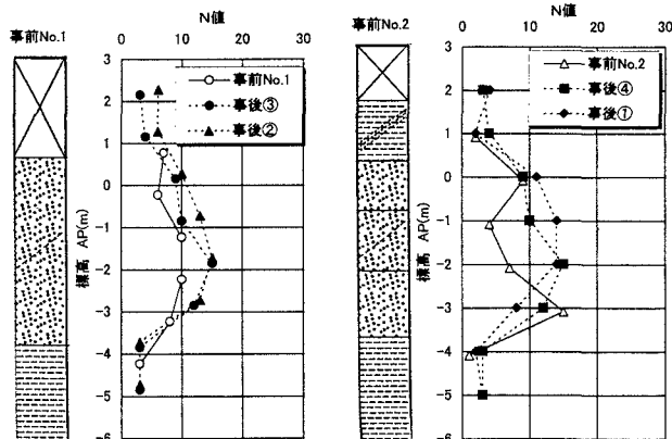
図-4 改良前後のN値の比較
