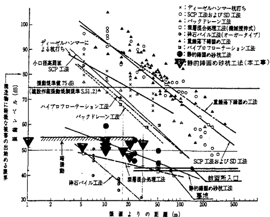
図-3 振動レベルの距離減衰 文献4)に一部加算
