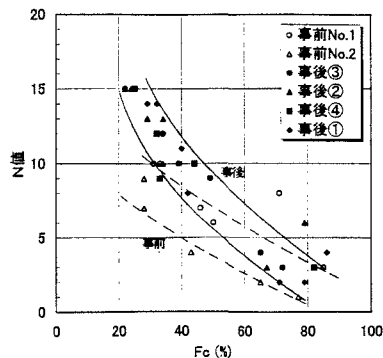
図-6 細粒分含有率とN値の関係
