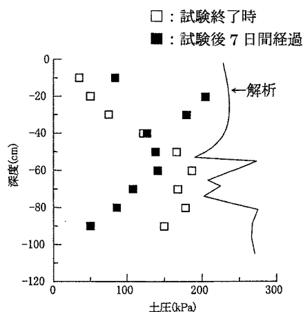
図 3 土圧に関する解析と実験結果の比較
