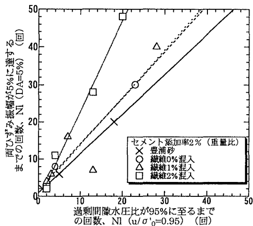
図4 DA=5%と過剰間隙水圧比が95%に至るまでの回数の違い
