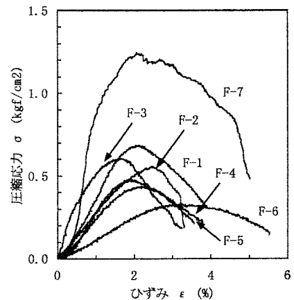
図4 応力—ひずみ曲線
