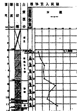
図1 土質柱状図
