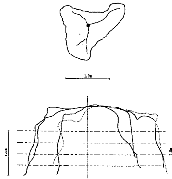
図-4 掘削による注入固化範囲の確認
