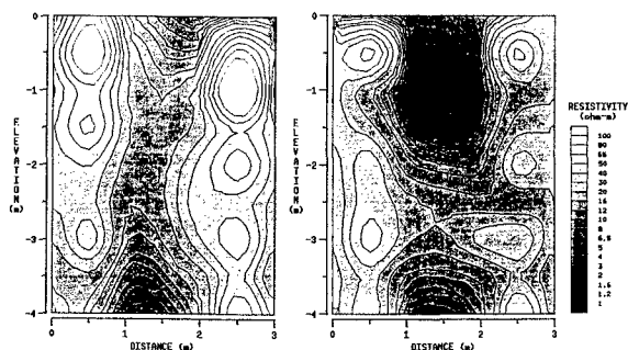
図-2 浸透注入部の比抵抗分布
