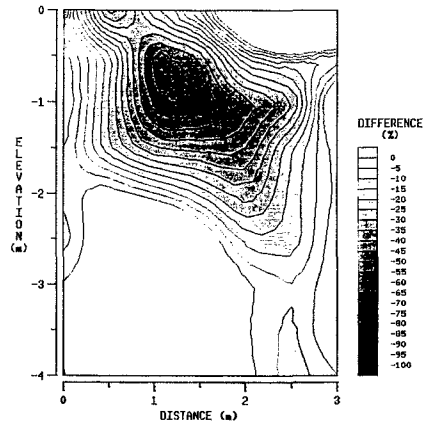
図-3 注入前後の比抵抗変化率(%)
