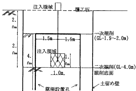
図-1 比抵抗トモグラフィ測定状況
