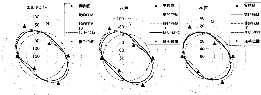
図2 軸力図
