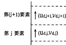
図4 排水部材内流れ
