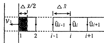
図2 地盤部の空間的離散化
