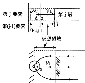
図3 排水部材内への流れ
