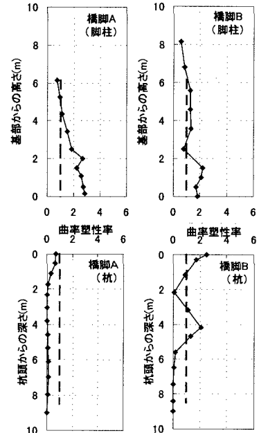
図-6 曲率塑性率分布
