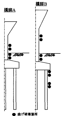
図-7 解析損傷箇所
