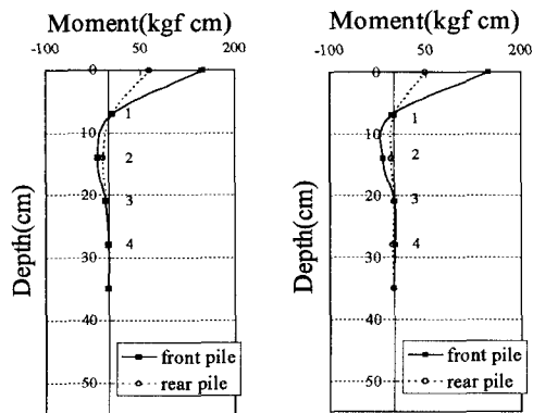
図-3 曲げモーメント分布
