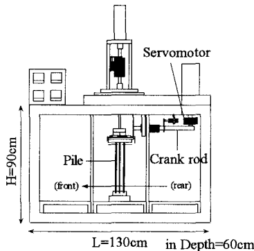
図-1 実験装置
