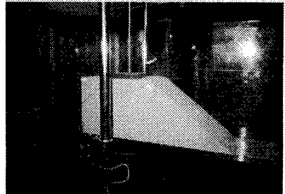
図1 実験状況（斜面崩壊）
