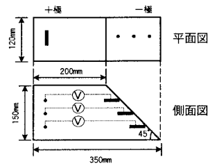
図2 電極配置例（V:電圧、A:電流）
