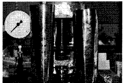
図3 実験状況（岩石破壊）
