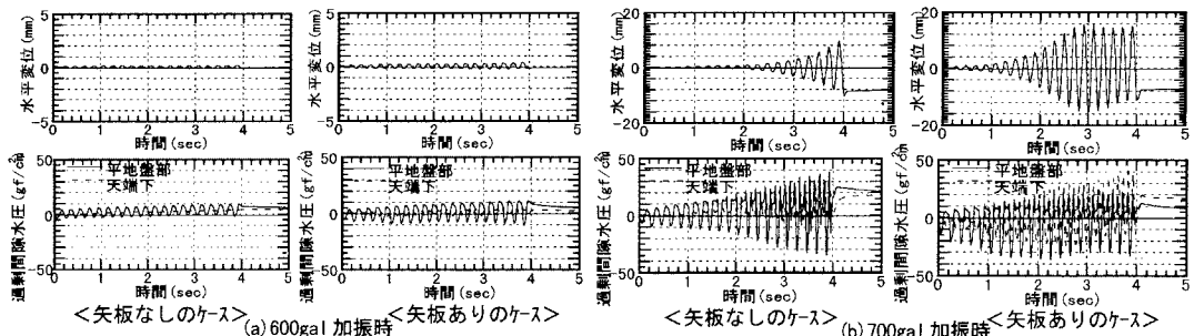
図2 矢板頭部(矢板なしのケースではのり肩位置)の水平変位と基礎地盤の過剰間隙水圧の経時変化
