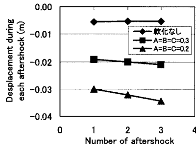
Fig.5 各余震毎の法尻の残留水平変位量.
