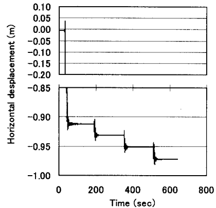
Fig.4 法尻の水平応答変位の時刻歴.
