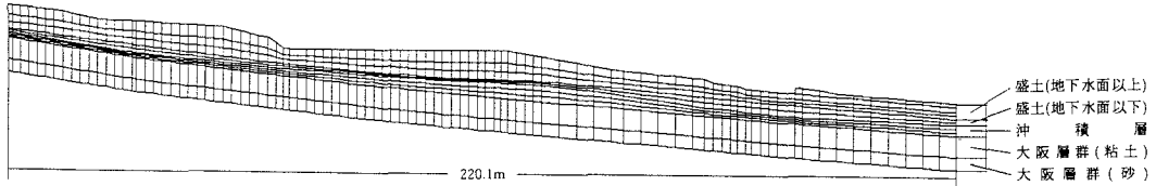
図-1 解析地盤モデル
