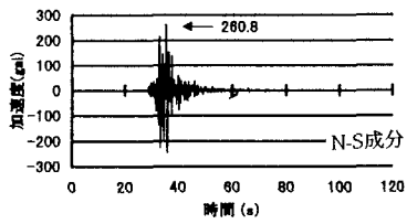
図-2 入力地震動
