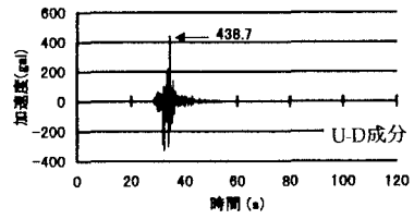
図-2 入力地震動
