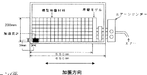
図 2.1 実験モデル
