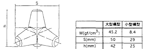
図-1 消波ブロック模型とサイズ
