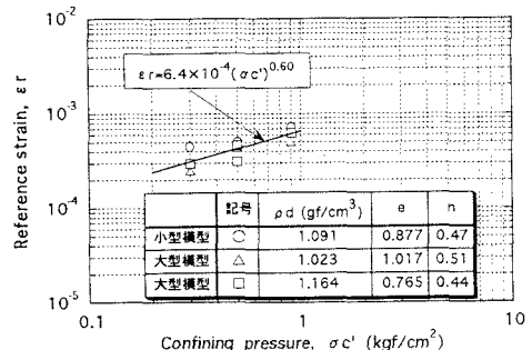
図-4 \varepsilon_r と拘束圧の関係
