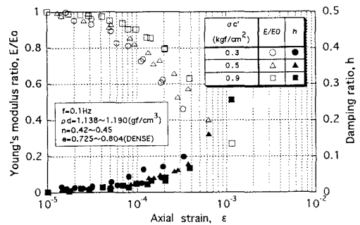
図-2 E/E_0, h \sim \varepsilon 関係の拘束圧依存性の代表例
