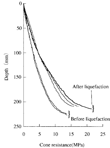
図-5 コーン抵抗値の深度方向分布
