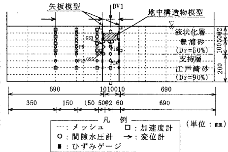
図1 実験模型
