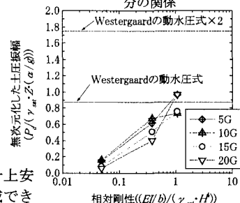
図8 矢板剛性とモーメント振動成分の関係
