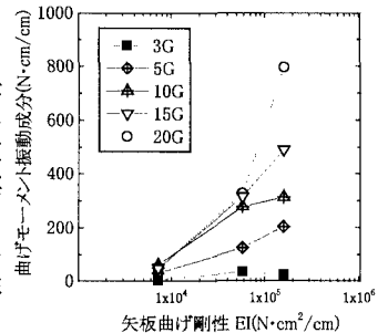
図6 矢板剛性とモーメント振動成分の関係
