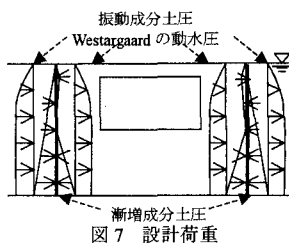
図7 設計荷重
