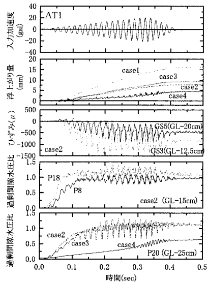
図2 時刻歴
