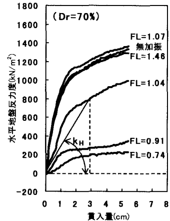
図-4 貫入量と水平地盤反力度
