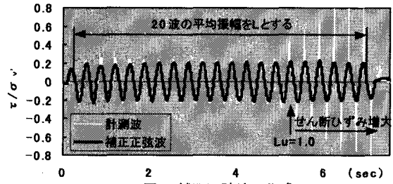
図-3 補正正弦波の作成
