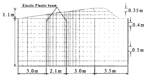
図-3 解析メッシュ
