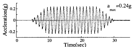
図-2 入力波形（TEST2）
