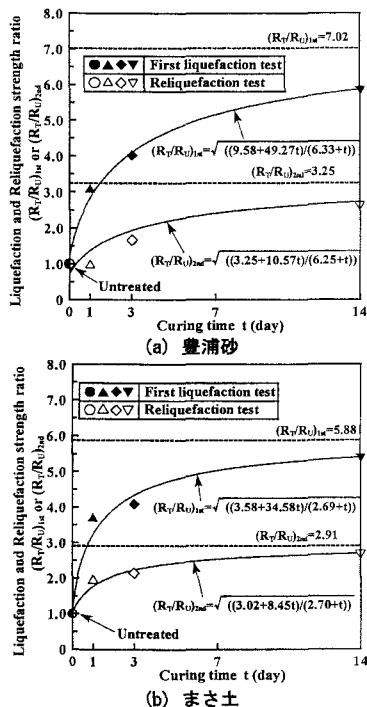
図-3 液状化強度比および再液状化強度比と養生日数との関係
