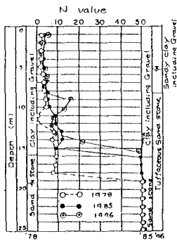
Fig. 3(b) 鷺ヶ丘団地BP-36N値分布
