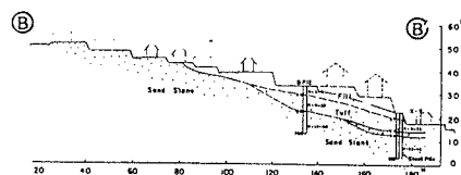
Fig.2(b) B-B' 断面図
