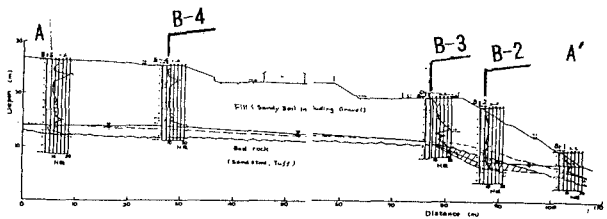
Fig. 6 A-A' 断面図
