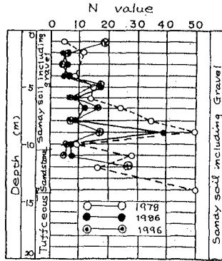
Fig. 7(b) 鷺ヶ谷団地B-3 N値分布
