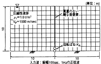
図1 解析モデル
