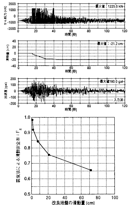
図8 改良地盤の滑動安全率と滑動量
