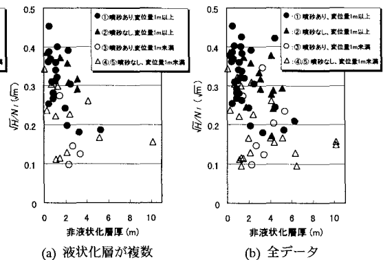
図3 \sqrt{H}/N_1 と液状化層上部の非液状化層厚の関係
