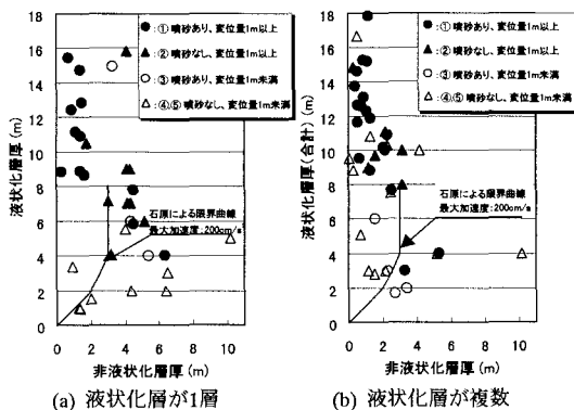
図2 液状化層厚と液状化層上部の非液状化層厚の関係
