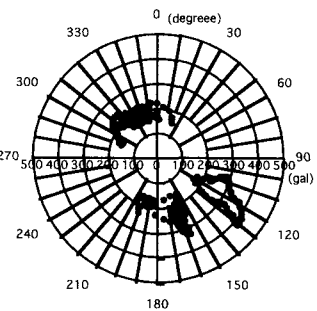
図-3 加速度の軌跡(150gal以上)
