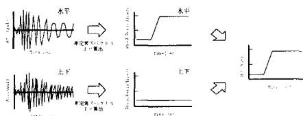
(b) 液状化発生時（表面波なし）
