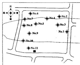
図-5 A地点小学校のボーリング位置図
