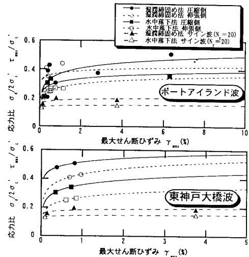
図4 応力比とせん断ひずみの関係
