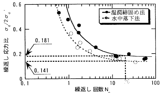
図2 液状化曲線
