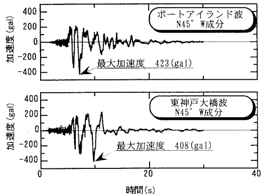
図1 加速度時刻歴
