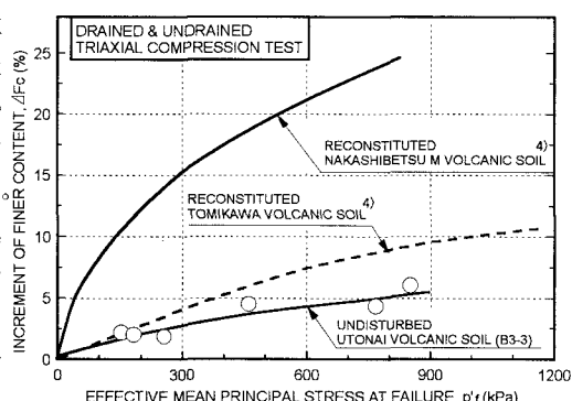
図-2 不攪乱及び再構成火山灰土の粒子破碎特性
