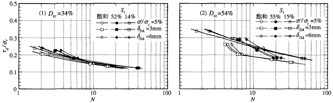
図-3 三隅砂における飽和度と繰返し強度の関係
