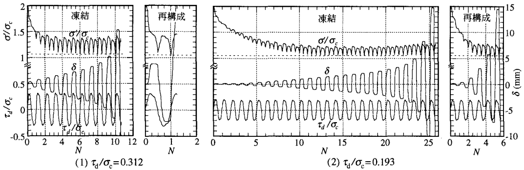
図-4 神戸砂凍結・再構成試料の \tau_d/\sigma_c , \delta , \sigma'/\sigma_c - N 関係の比較
