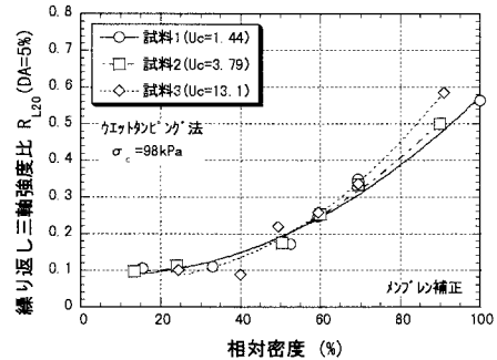
図3 相対密度と繰り返し三軸強度比 R_{L50} の関係
