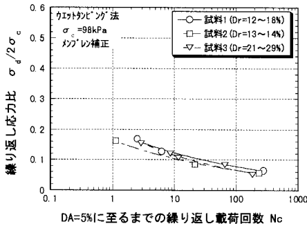
図2 砂礫材料の液状化試験結果 ( Dr \approx 10\% )
