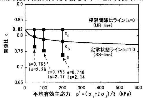
図 2 I_s の定義
