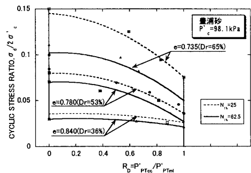
図4 CSR, N_{1\%} が強度低下に及ぼす影響
