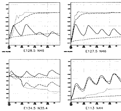
図3 W_1, W_2 の control-run との差 (経時変化)
