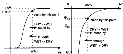
図1 土壌水分の特機点
