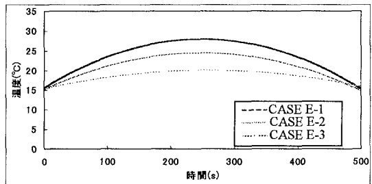
図-4 実験結果 (x=40cm, y=20cm)
