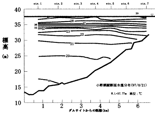
図-3 水温縦断面分布(97/8/21)
