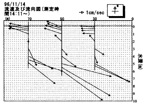
図-7 stn.6における流向・流速図
