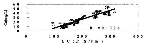
図-2 EC と Ca の関係
