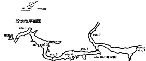
図-1 小野湖(厚東川ダム貯水池)
