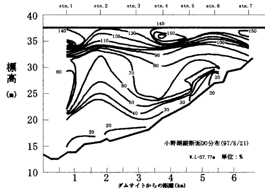
図-6 DO 縦断面分布(97/8/21)
