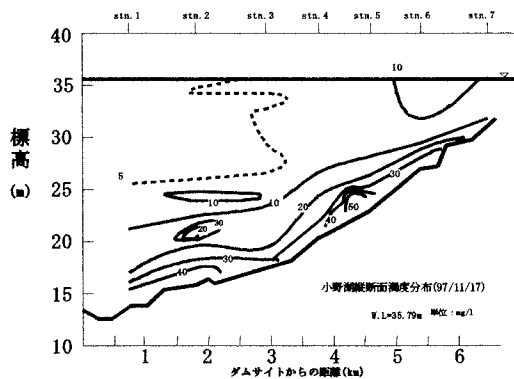
図-5 濁度縦断面分布(97/11/17)
