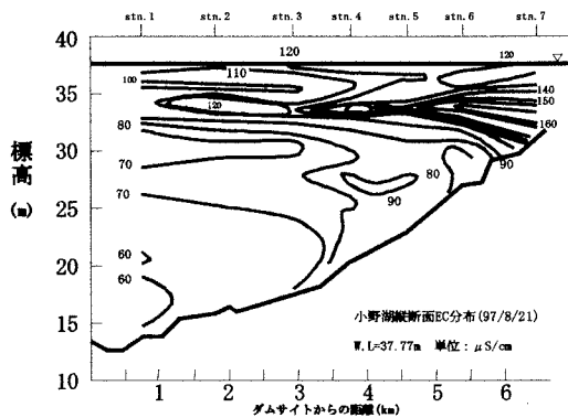
図-4 EC 縦断面分布(97/8/21)
