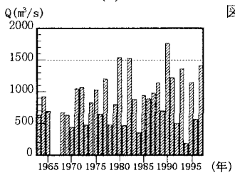
図-5 白川年最大流量経年変化
