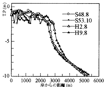
図-2 滞筋部の縦断形状
