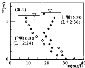
図-8 浮遊物質濃度の鉛直分布
