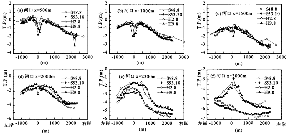
図-4 白川干潟地形の横断形状
