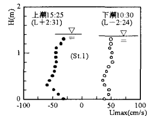
図-7 主流速の鉛直分布
