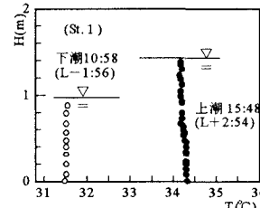
図-10 水温の鉛直分布
