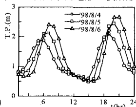
図-6 白川河口水位の時系列
