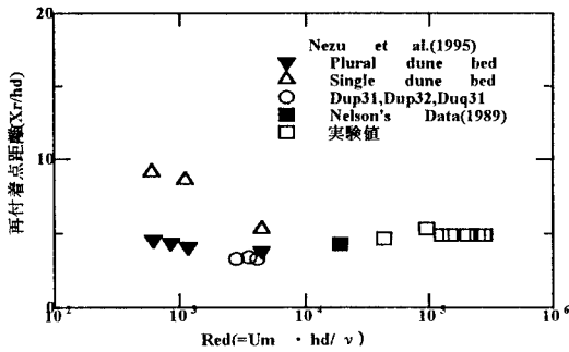
図-3 再付着点距離
