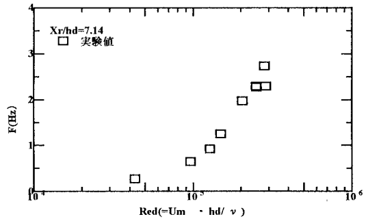
図-5 流速変動の卓越周波数
