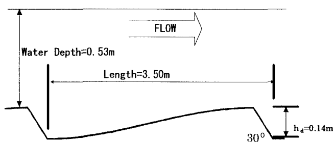
図-1 河床模型図
