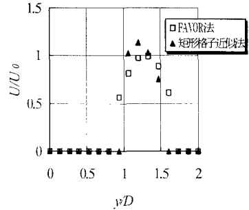
図-8 断面流速分布 (ケース 3)
