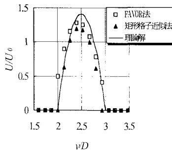
図-7 断面流速分布 (ケース 2)
