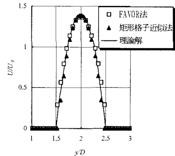
図-6 断面流速分布 (ケース 1-(b))
