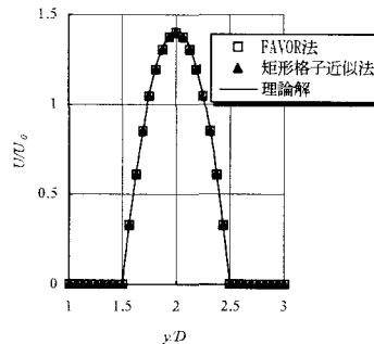
図-5 断面流速分布 (ケース 1-(a))
