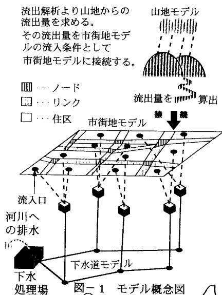
図-1 モデル概念図
