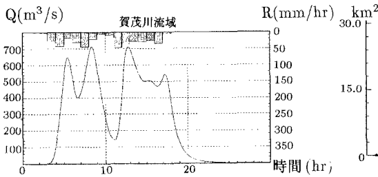
図-3 降雨量と流出流量
