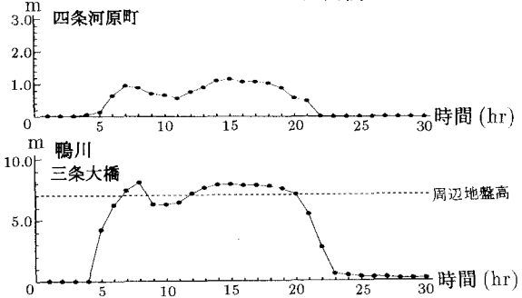
図-6 浸水深ならびに水深の時間的变化
