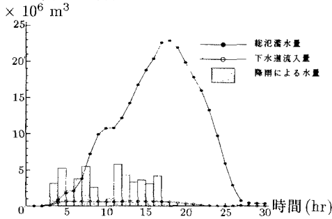
図-5 氾濫水量と下水道流入量
