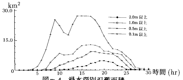
図-4 浸水深別氾濫面積
