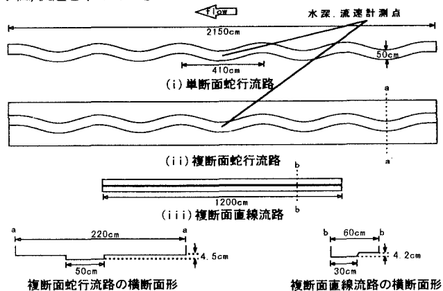
図-1 実験水路、及び水深、流速計測点
