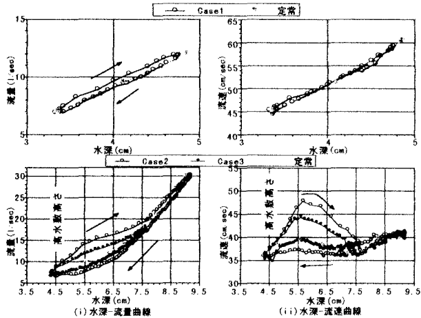
図-3 水深-流量、及び水深流速曲線
