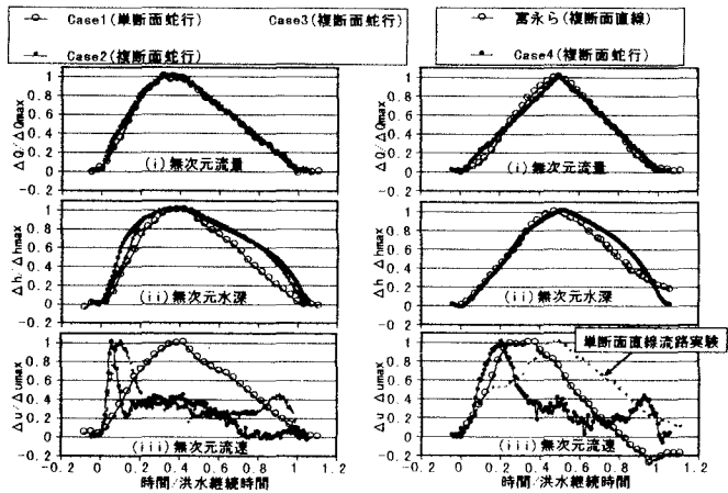
図-4 複断面蛇行流路と単断面蛇行流路の洪水流出特性
