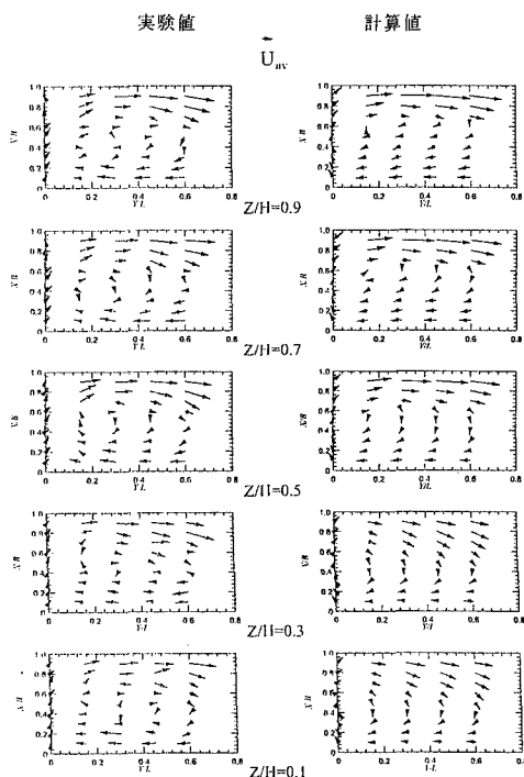
図-2 数値計算値と実験値の比較
