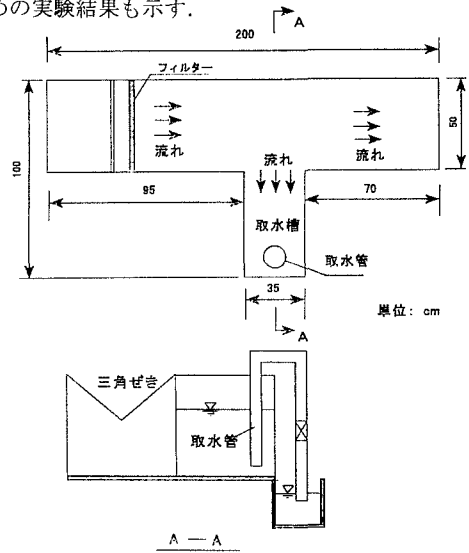
図-1 実験水槽と取水口模型
