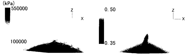
図2 初期物性値（せん断剛性）
