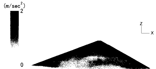
図5 最大加速度分布（三次元解析結果）
