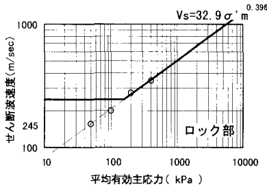
図4 セン断波速度と平均有効主応力の関係
