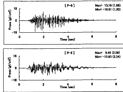
図－４ 600gal加振時の間隙水圧の時刻歴 （U字谷模型の上下流方向加振）
