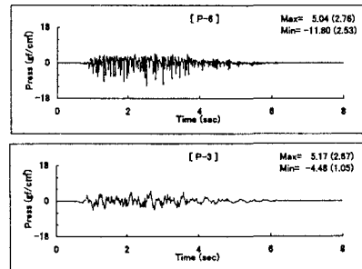
図－６ 600gal加振時の間隙水圧の時刻歴 （V字谷模型の上下流方向加振）
