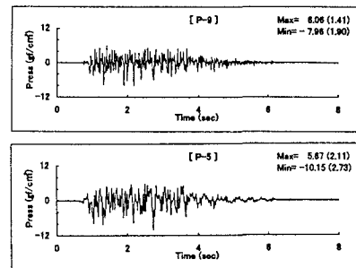
図－５ 600gal加振時の間隙水圧の時刻歴 （U字谷模型のダム軸方向加振）
