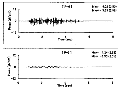
図－７ 600gal加振時の間隙水圧の時刻歴 （V字谷模型のダム軸方向加振）
