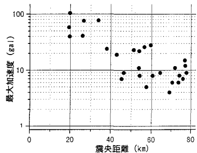
〈図-3〉 震央距離 距離減衰
