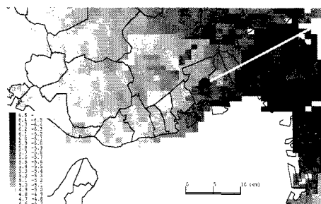
図2 堆積地盤上における計測震度分布(破壊開始点は断層西端)
